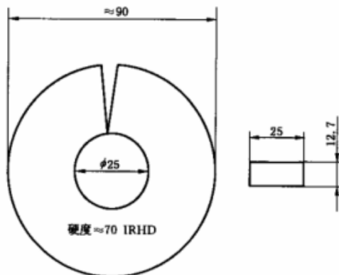
图 A.2 橡胶缓冲垫
